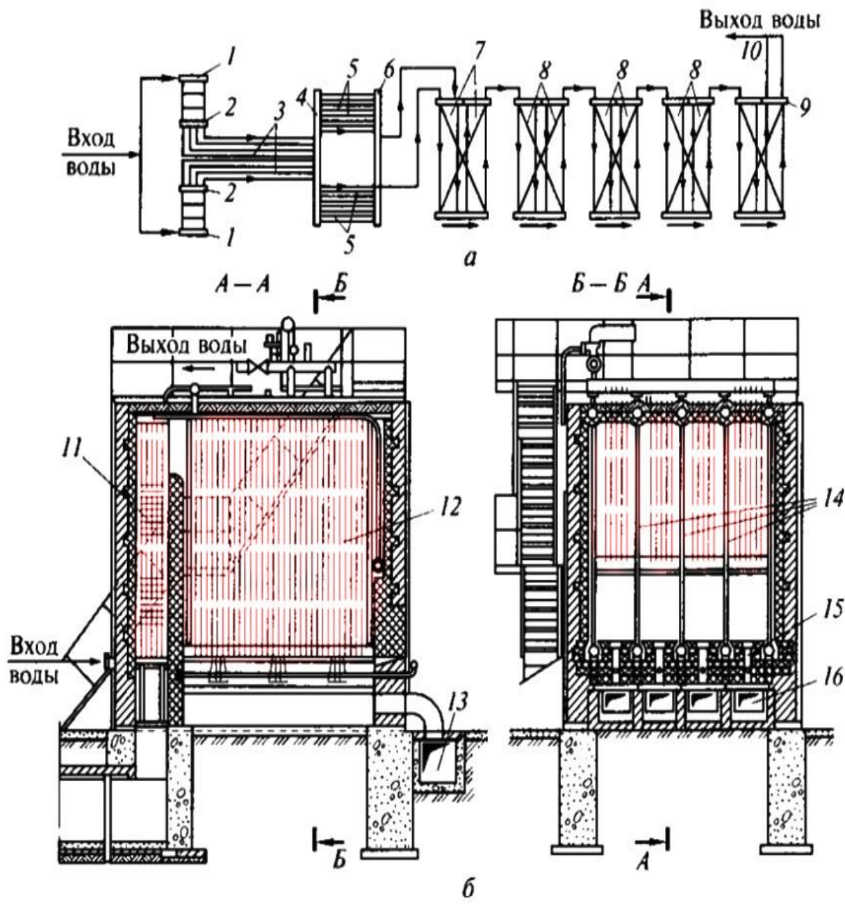
Рис. 3. Схема работы теплового оборудования
